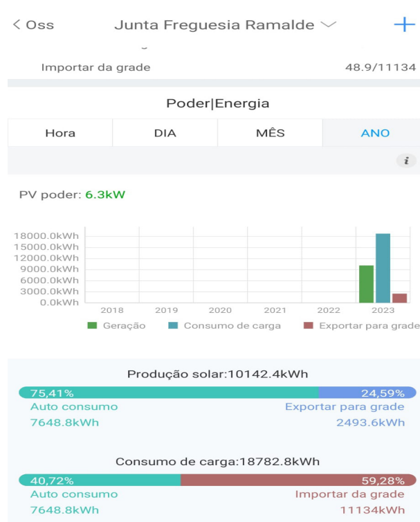
Figura 41 - Níveis de energia dos painéis fotovoltaicos do edifício sede da Junta de Freguesia de Ramalde.
